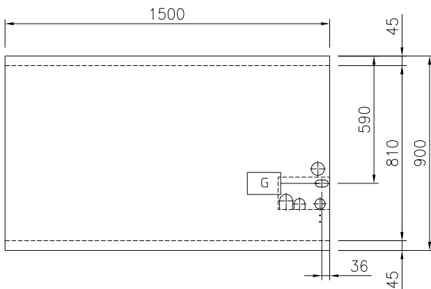
Boven aanzicht
