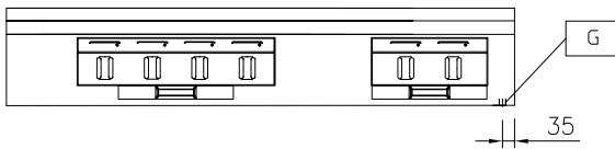
Front aanzicht
